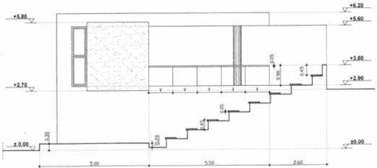
ΟΨΗ - ΤΟΜΗ Α-Α
